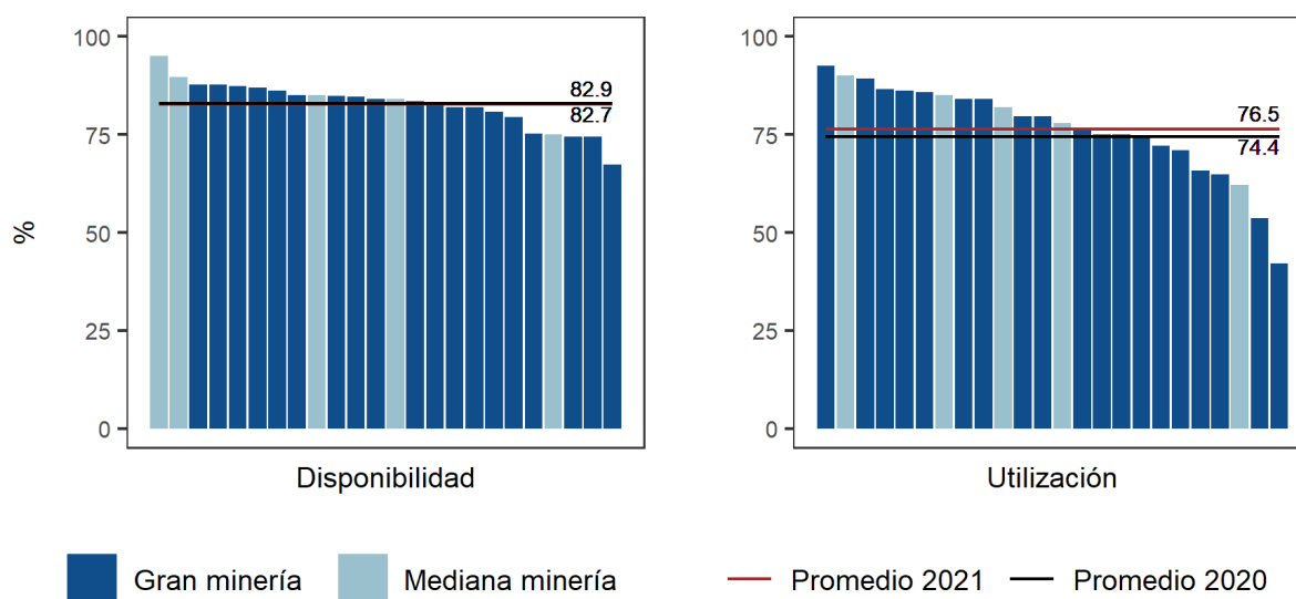
Figura 14: Indicadores de productividad del activo transporte en mina rajo, año 2021.
