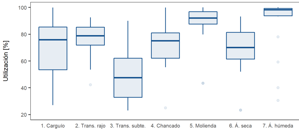
Figura 21: Resumen de indicadores de utilización, año 2021.
