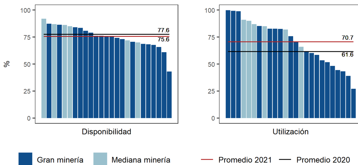
Figura 13: Indicadores de productividad del activo carguío en mina rajo, año 2021.
