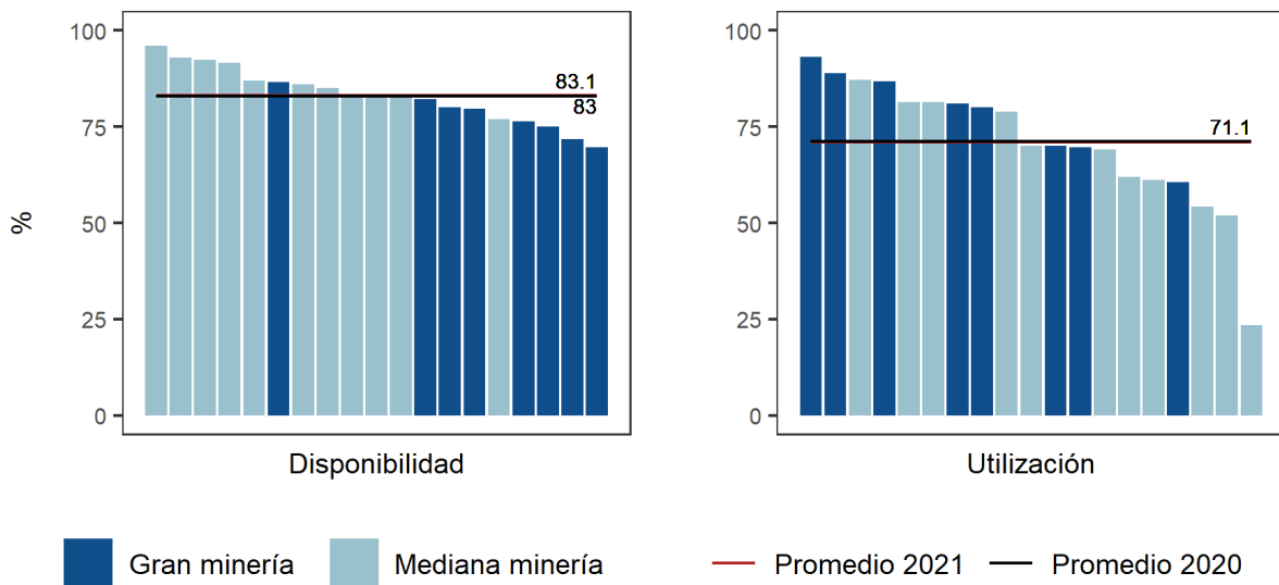
Figura 18: Indicadores de productividad del área seca en planta hidrometalúrgica, año 2021.
