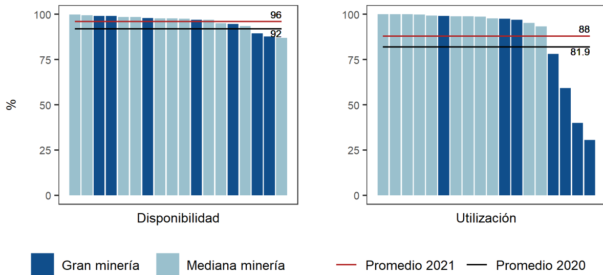
Figura 19: Indicadores de productividad del área húmeda en planta hidrometalúrgica, año 2021.
